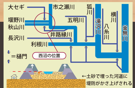
天井川のできる仕組みと周辺の河川の様子
