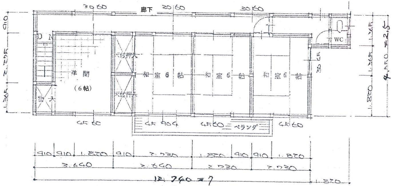
2階 平面図
